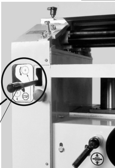
C - Piktogram spínání páky pohonu protahu.
